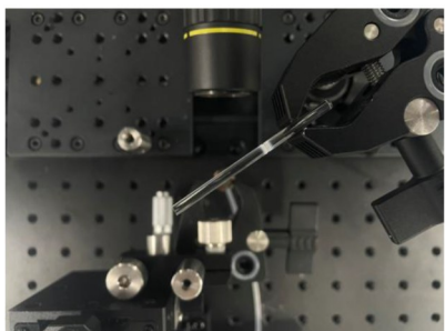
(b) 微棒腔加热装置的俯视图
