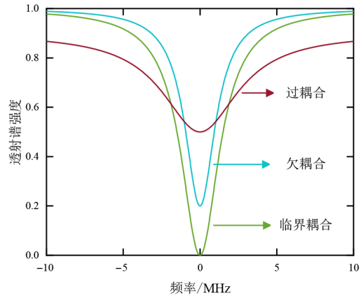
图1 欠耦合、过耦合、临界耦合三种耦合状态下微腔透射谱强度图
