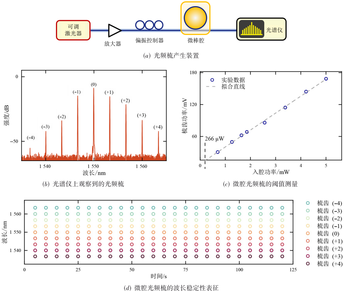
图6 基于二氧化硅微棒腔产生的微腔光频梳
