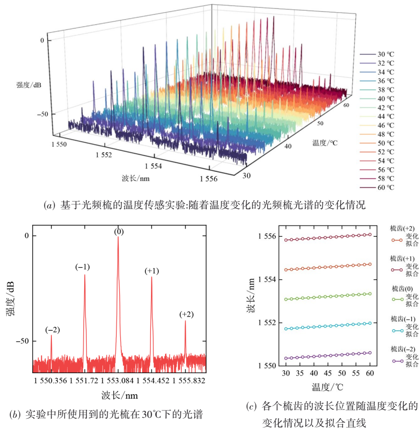
图7 基于光频梳的温度传感实验
