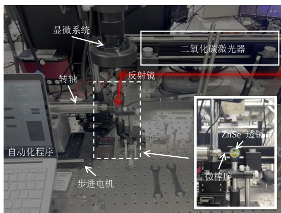
图2 二氧化硅微棒腔的制备装置图
