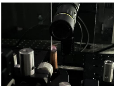
(a) 氢焰发生装置
