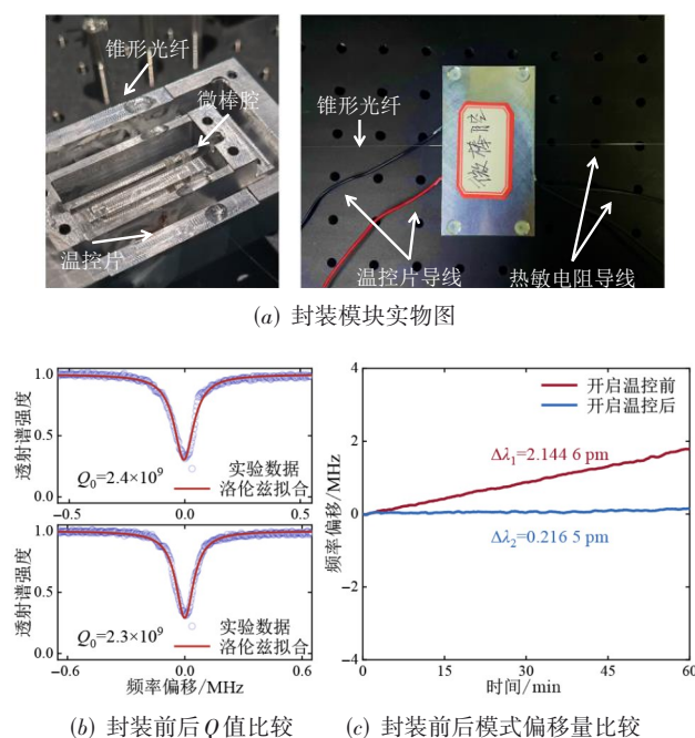
图5 微腔封装及性能表征
